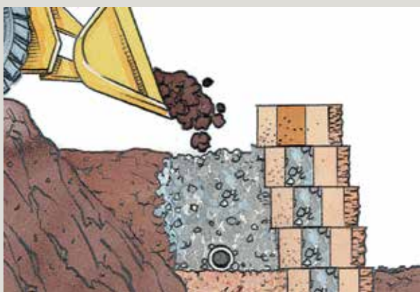
7 DRENERINGSMASSE*
