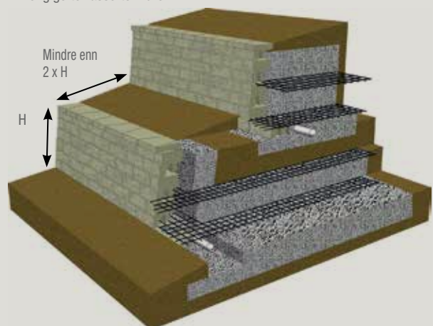
Avhengige terrasste murer
