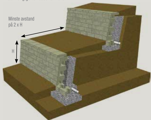
Uavhengige terrasste murer
