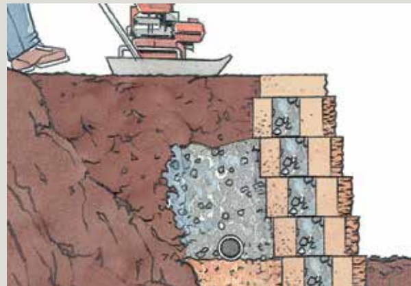
8 KOMPRIMERING
